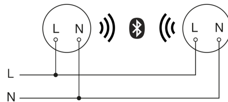
aansluitschema master/master
